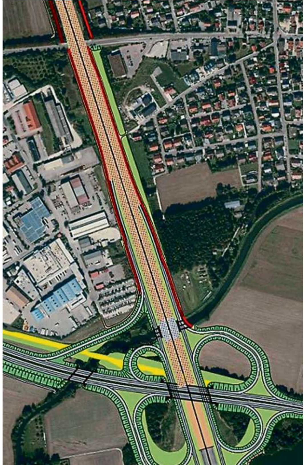
Planungsentwurf der Autobahnanschlussstelle Manching als Kleeblatt mit Lärmschutzwall (rote Linien) entlang der Autobahn Richtung Norden. Zudem kommt Flüsterasphalt auf die A9 vor Manching (orange gepunktet).
