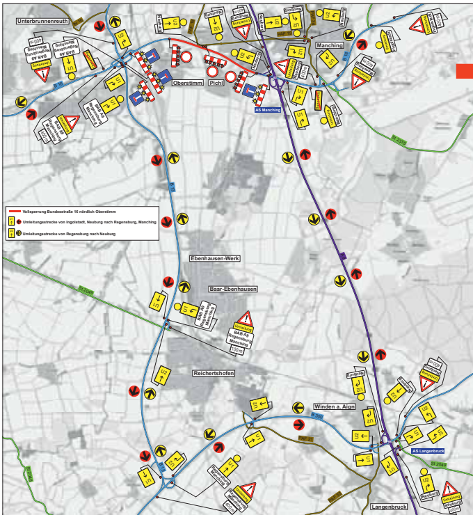
Umleitungsplan Vollsperrung B16 westlich der A9
