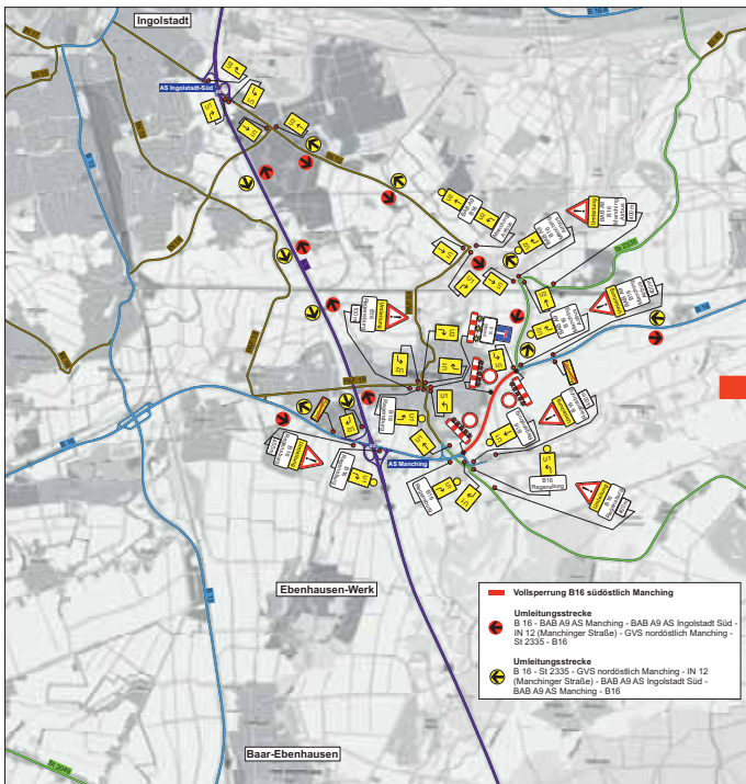
Umleitungsplan Vollsperrung B16 östlich der A9
